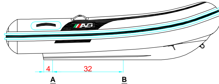
LONGITUDINAL PROFILE VISTA LATERAL
